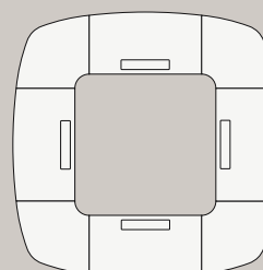
16 personnes (330 x 330 cm) Sans TA : Réf. ICR 25 Avec TA : Réf. ICR 25 TA
