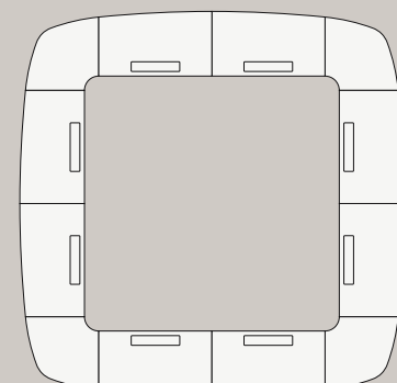
24 personnes (476 x 476 cm) Sans TA : Réf. ICR 28 Avec TA : Réf. ICR 28 TA
